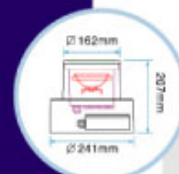
Model: ODL-162SQ(AR-111)
