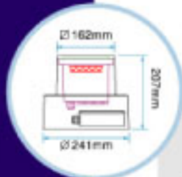
Model: ODL-162SQ(MD-12)
